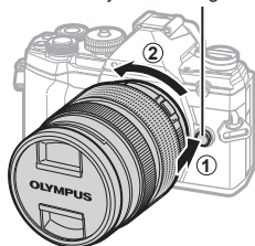
Objektívkioldó gomb
