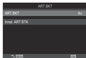
ART BKT-innstillingsskjerm
