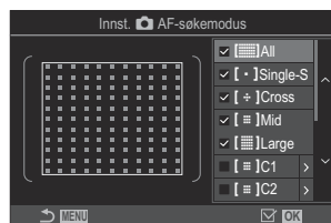
Innstillingsskjermbildet AF-søkemodus
