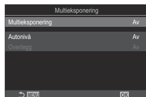
Innstillingsskjermbildet «Multieksponering»
